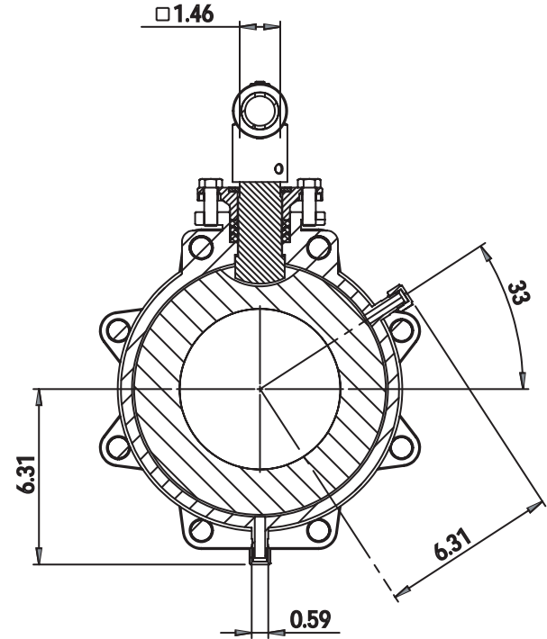
SECTION D-D
