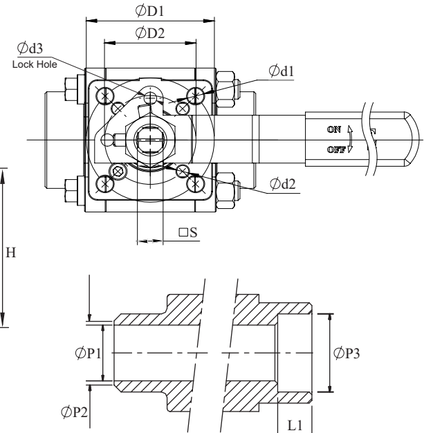
Butt Weld (Sch.40) // Socket Weld
